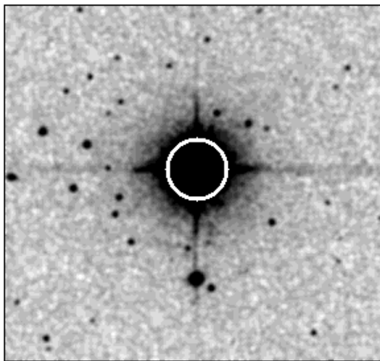
SAO 73156 J = 4.85
