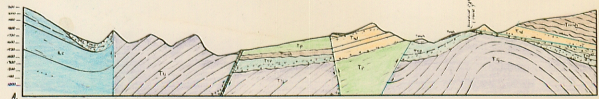
SECTION A-B
