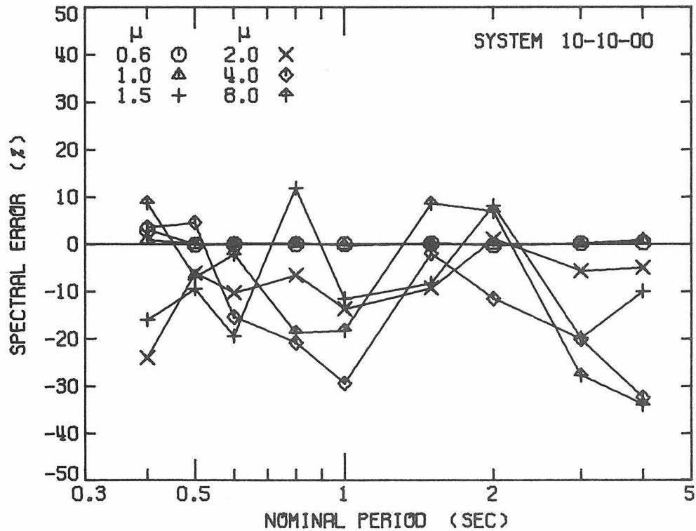
Figure 5.13b. Spectral Error - El Centro Spectra.
