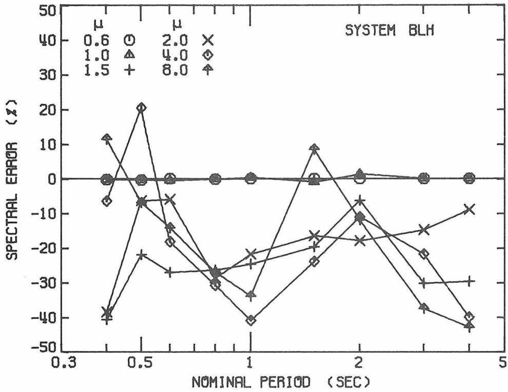
Figure 5.11a. Spectral Error - El Centro Spectra.
