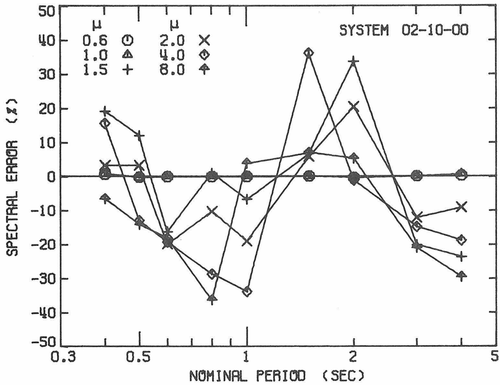
Figure 5.13a. Spectral Error - El Centro Spectra.
